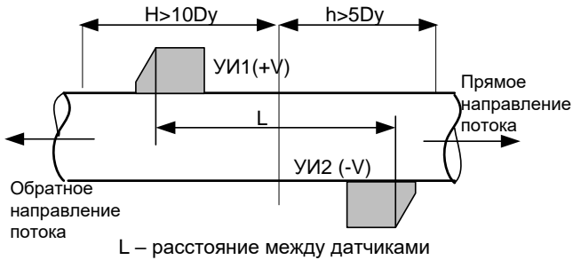
Вариант Z (двусторонняя установка УИ1 и УИ2)
