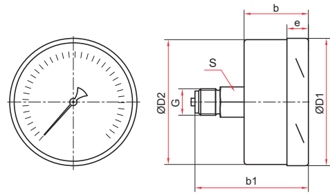
Осевое присоединение (KM-22)
