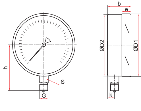
Радиальное присоединение (KM-31)
