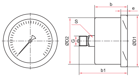
Осевое присоединение (KM-12)
