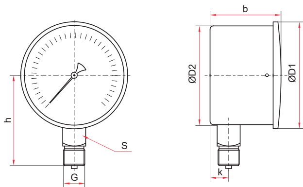
Радиальное присоединение (KM-11)
