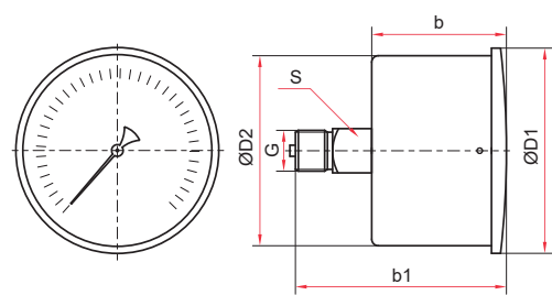
Осевое присоединение (KM-11)
