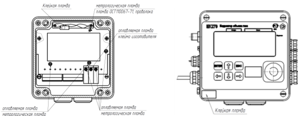
Рис. 3 Расположение пломб
