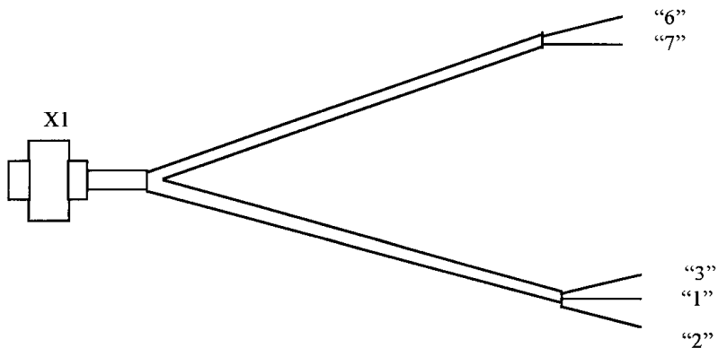
Рисунок Д.1 – Монтаж кабеля «ППР7-ИП7»
