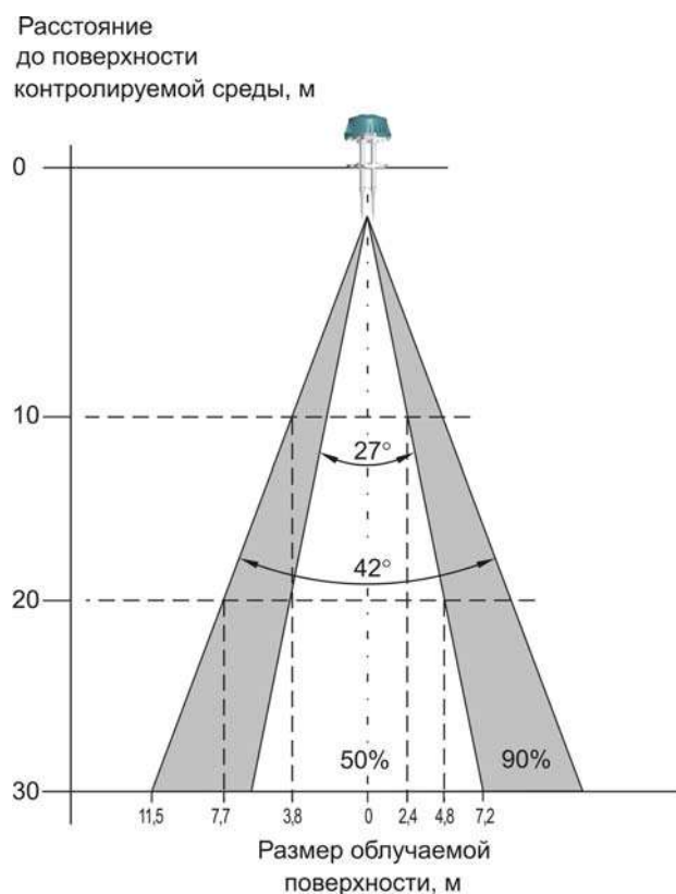
Рисунок 20 - Диаграмма направленности уровнемера исполнений БАРС 322МИ-07, БАРС 332МИ-07
