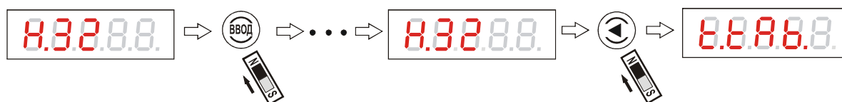
Рисунок 62 - Запись в память уровнемера 32 точек тарифовочной таблицы
