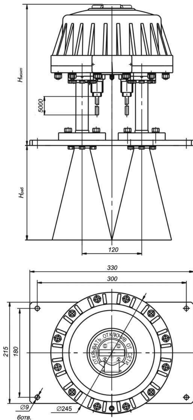
Рисунок 6 - Габаритные и установочные размеры уровнемера исполнений БАРС 322МИ-01, БАРС 322МИ-02, БАРС 332МИ-01
