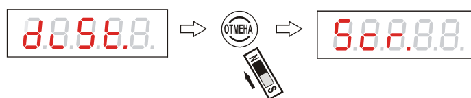
Рисунок 73 - Выход из подраздела выбора режима отображения
