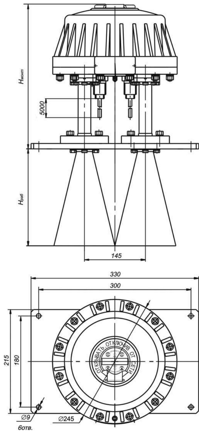
Рисунок 7 - Габаритные и установочные размеры уровнемера исполнения БАРС 332МИ-02
