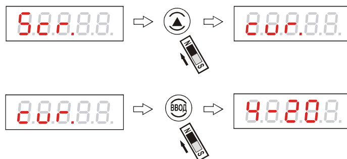
Рисунок 74 - Выбор диапазона токового выхода
