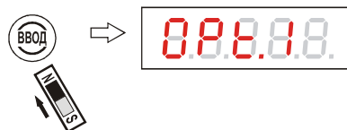
Рисунок 30 - Вход в режим программной настройки уровнемера
