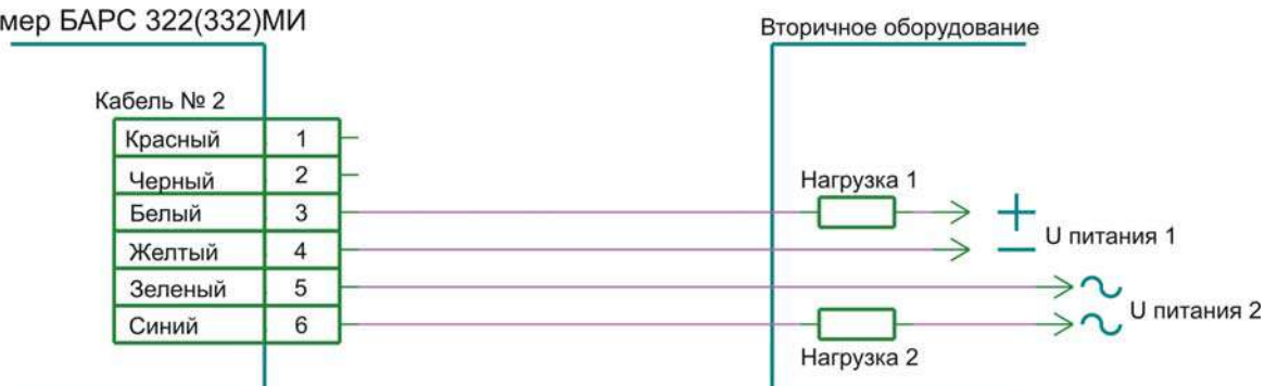
Рисунок Б.3 – Пример подключения цепей релейных выходов
