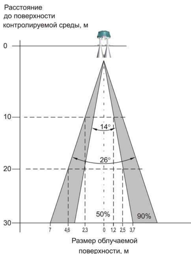
Рисунок 19 - Диаграмма направленности уровнемера исполнений БАРС 332МИ-02, БАРС 332МИ-04, БАРС 332МИ-06
