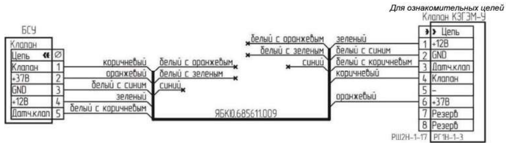
Рисунок А.4 – Схема подключения клапана КЗГЭМ-У с разъемом RJ1H-1-3.
