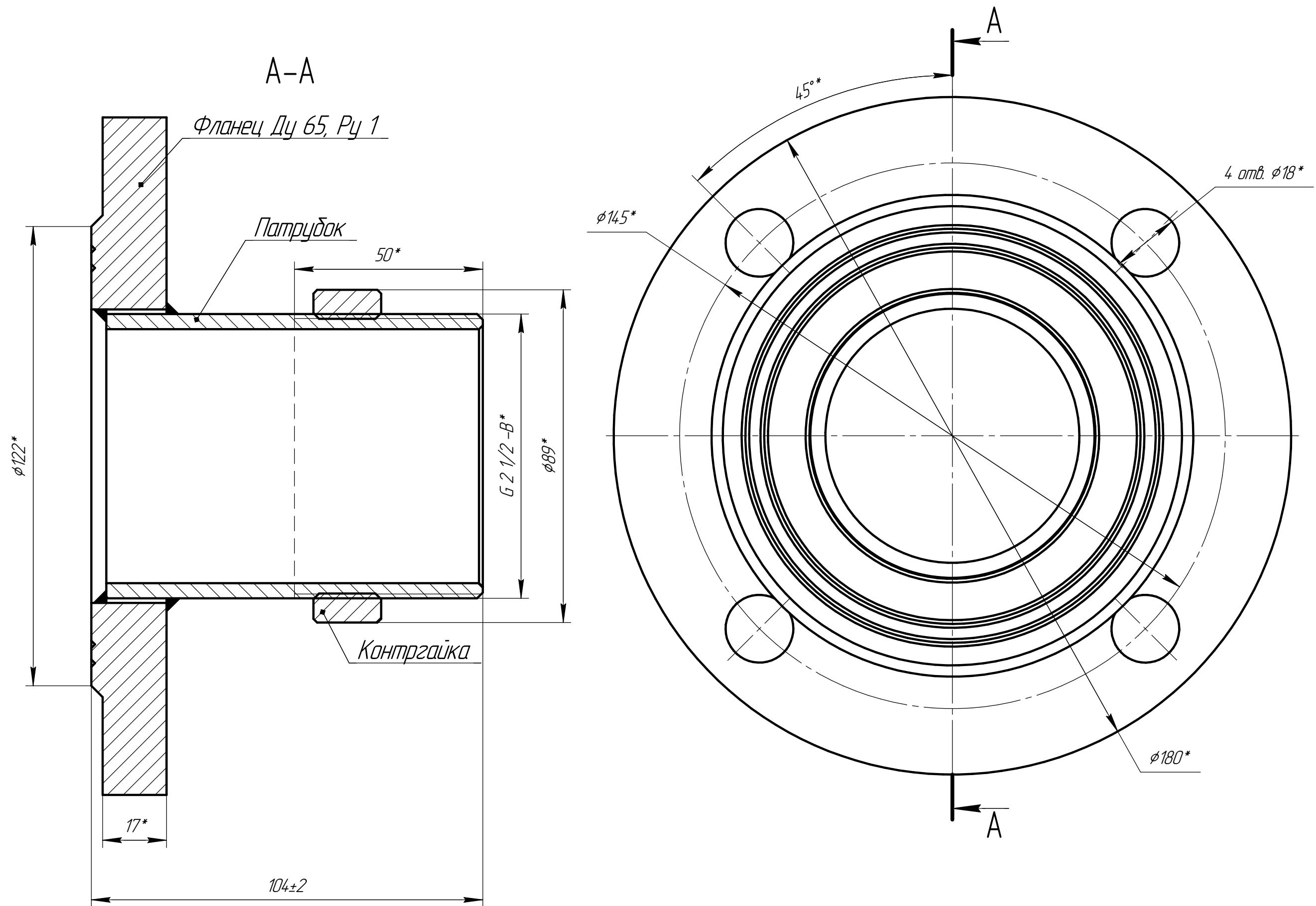
Узел фланцевый DN-65
