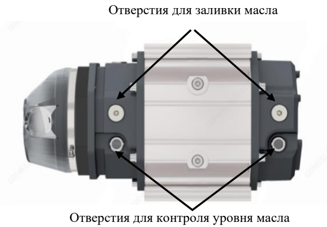
Рисунок 16. Заливка и контроль уровня масла при установке счетчика G10-G400 на вертикальном участке трубопровода
