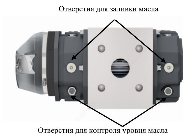
Рисунок 15. Заливка и контроль уровня масла при установке счетчика G10-G400 на горизонтальном участке трубопровода
