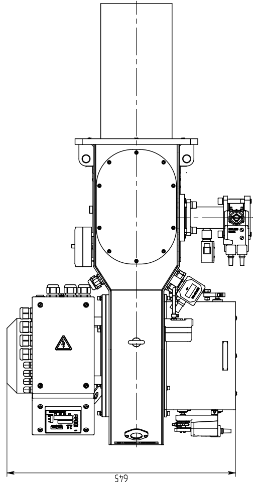
Рисунок А.2. Габаритные и присоединительные размеры горелки
