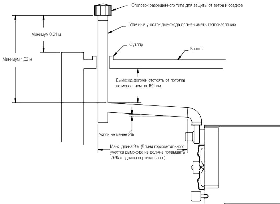
Схема расположения вертикального дымохода
