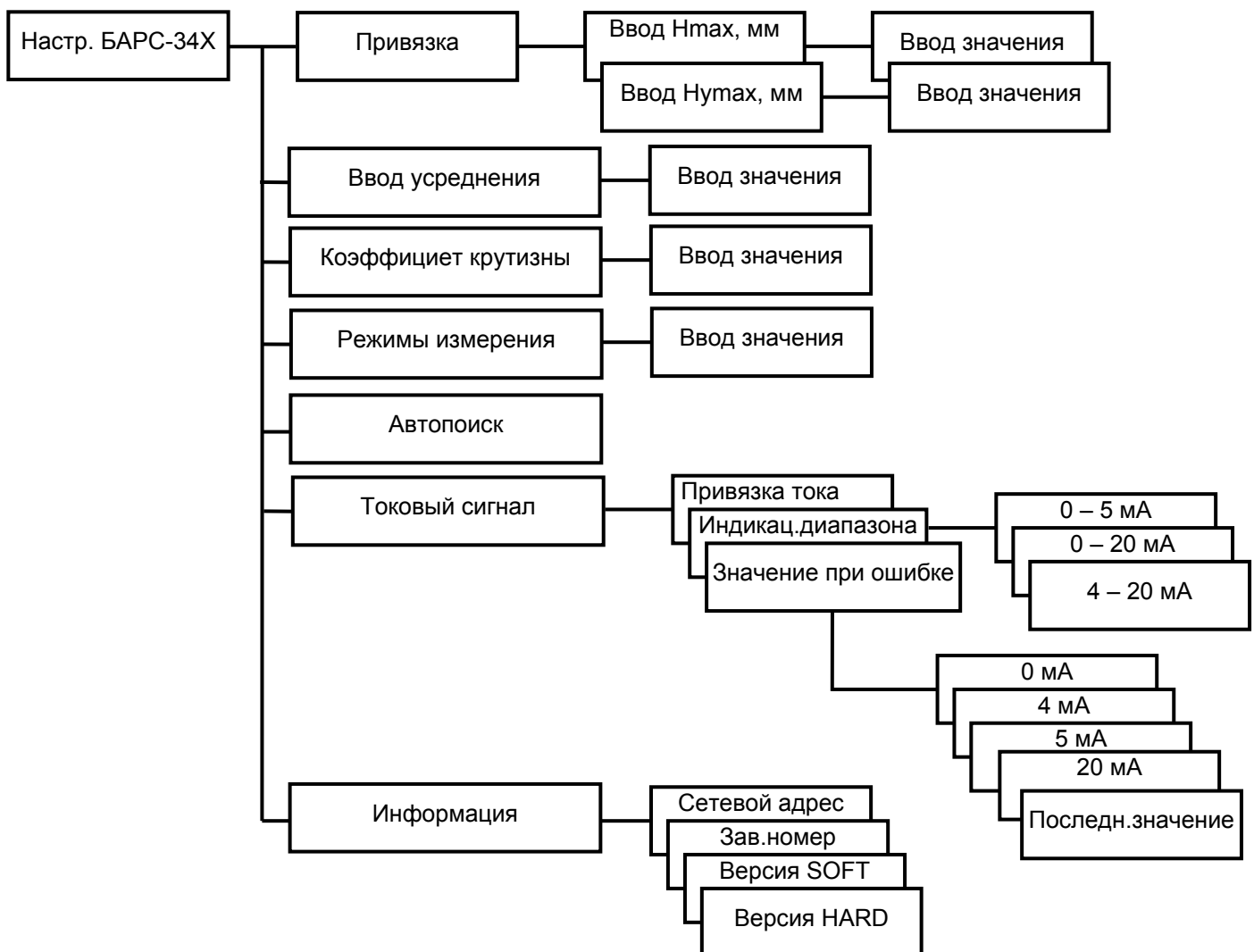
Рисунок М.1 – Меню настроек радиоволнового преобразователя уровня БАРС 341И.ХХ
