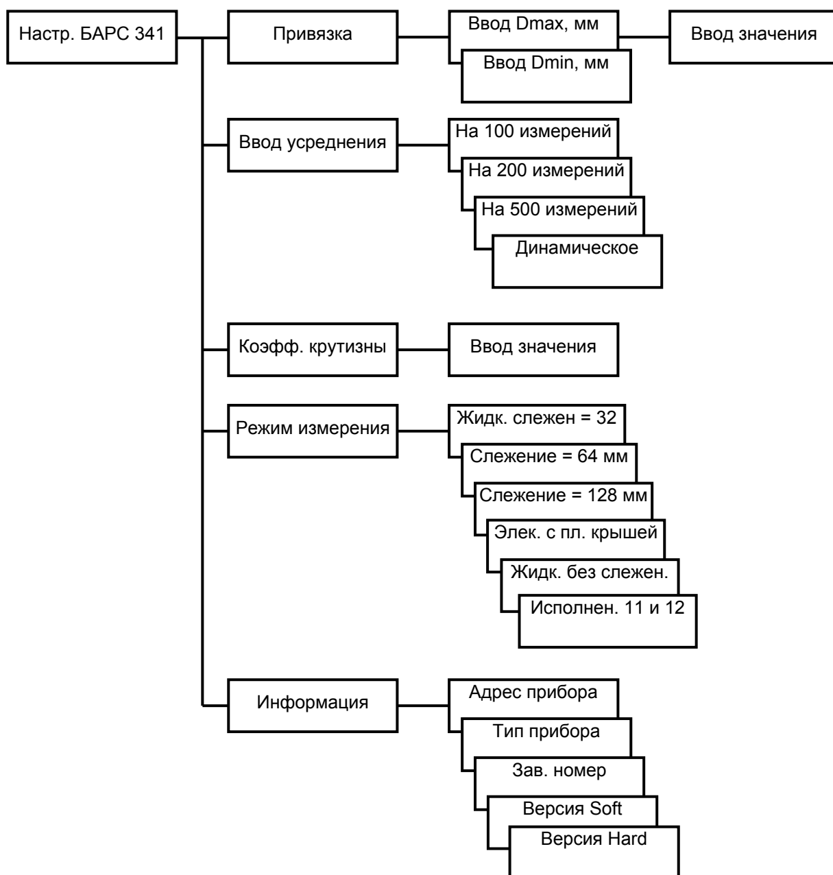
Рисунок Ж.3 – Схема меню настроек прибора при работе с радиоволновым преобразователем уровня БАРС 341И.ХХ
