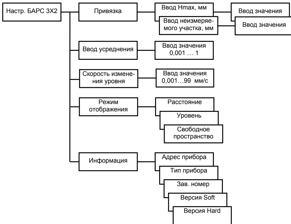
Рисунок И.2 – Схема меню настроек при работе прибора с радиоволновыми уровнемерами БАРС 322МИ-XX и БАРС 332МИ-XX
