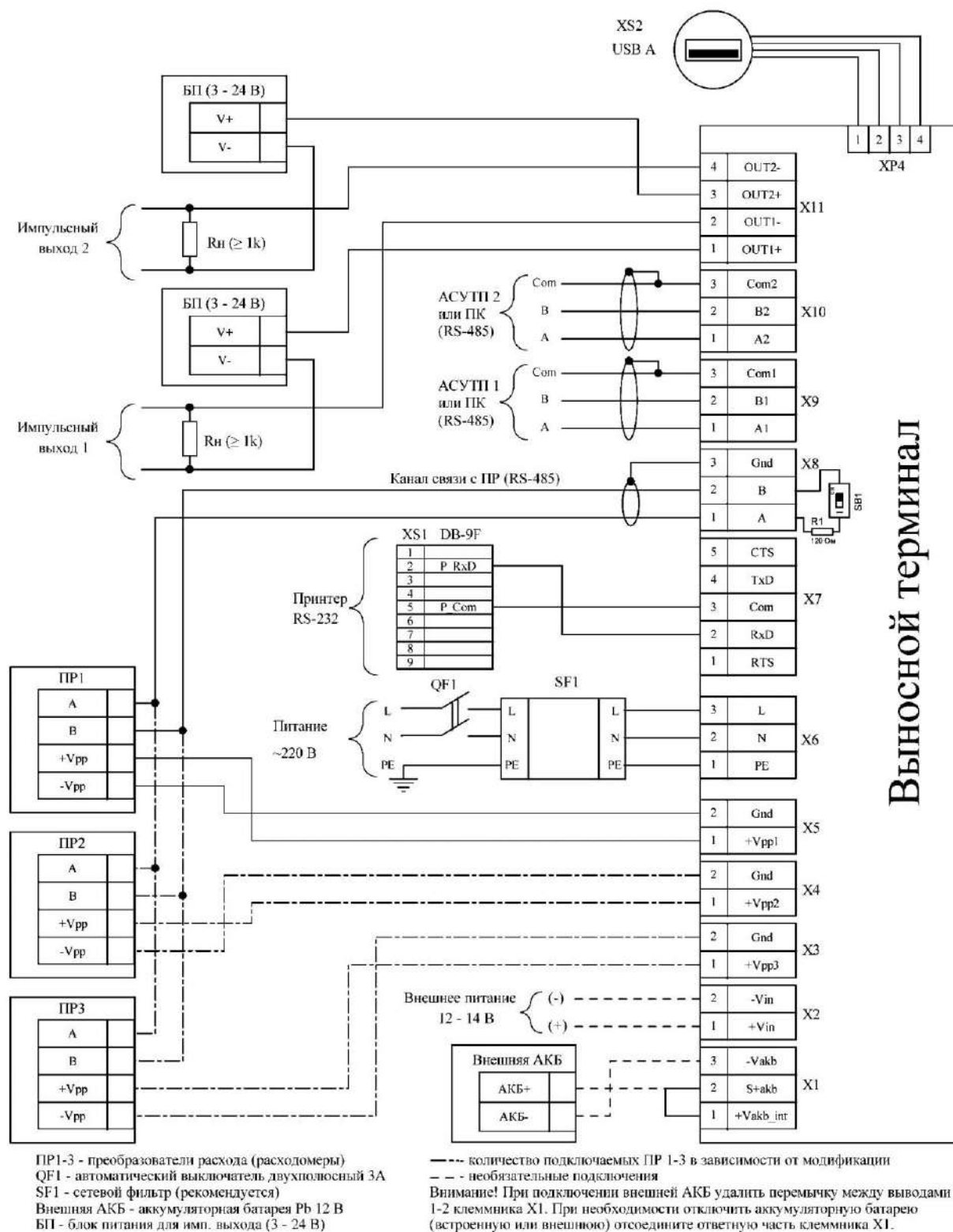
Рисунок Е.1 – Схема электрическая соединений ВТ
