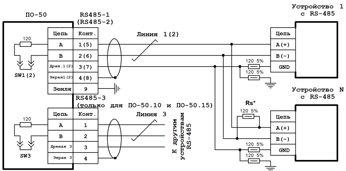
Рисунок 6 Схема подключения экранированной линии RS-485 с дренажным проводом
