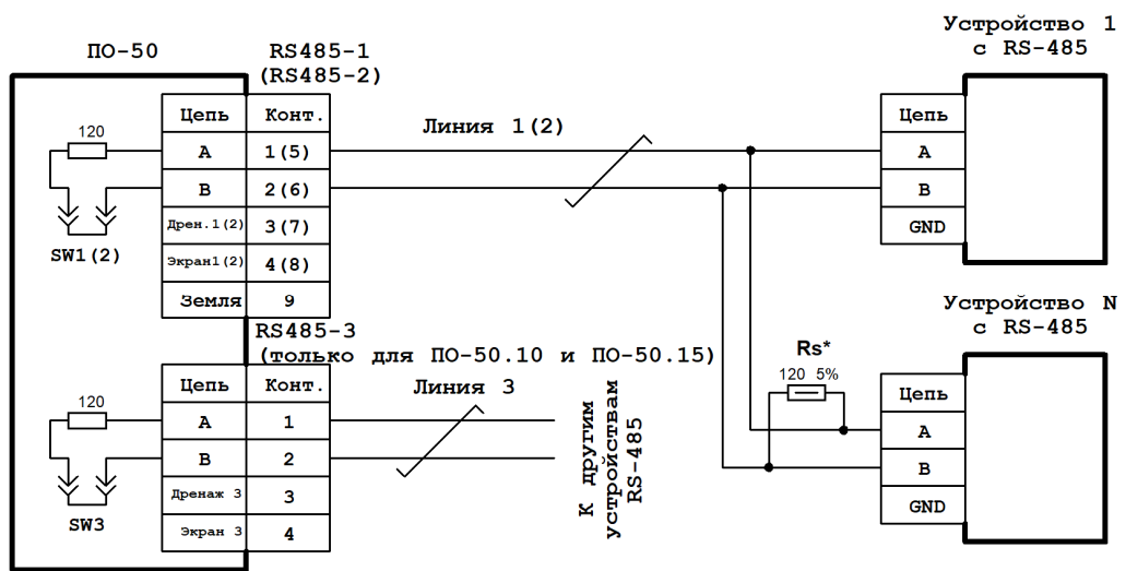
Рисунок 5 Схема подключения линии RS-485
