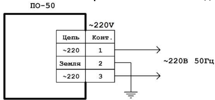
Рисунок 4 Схема подключения питания
