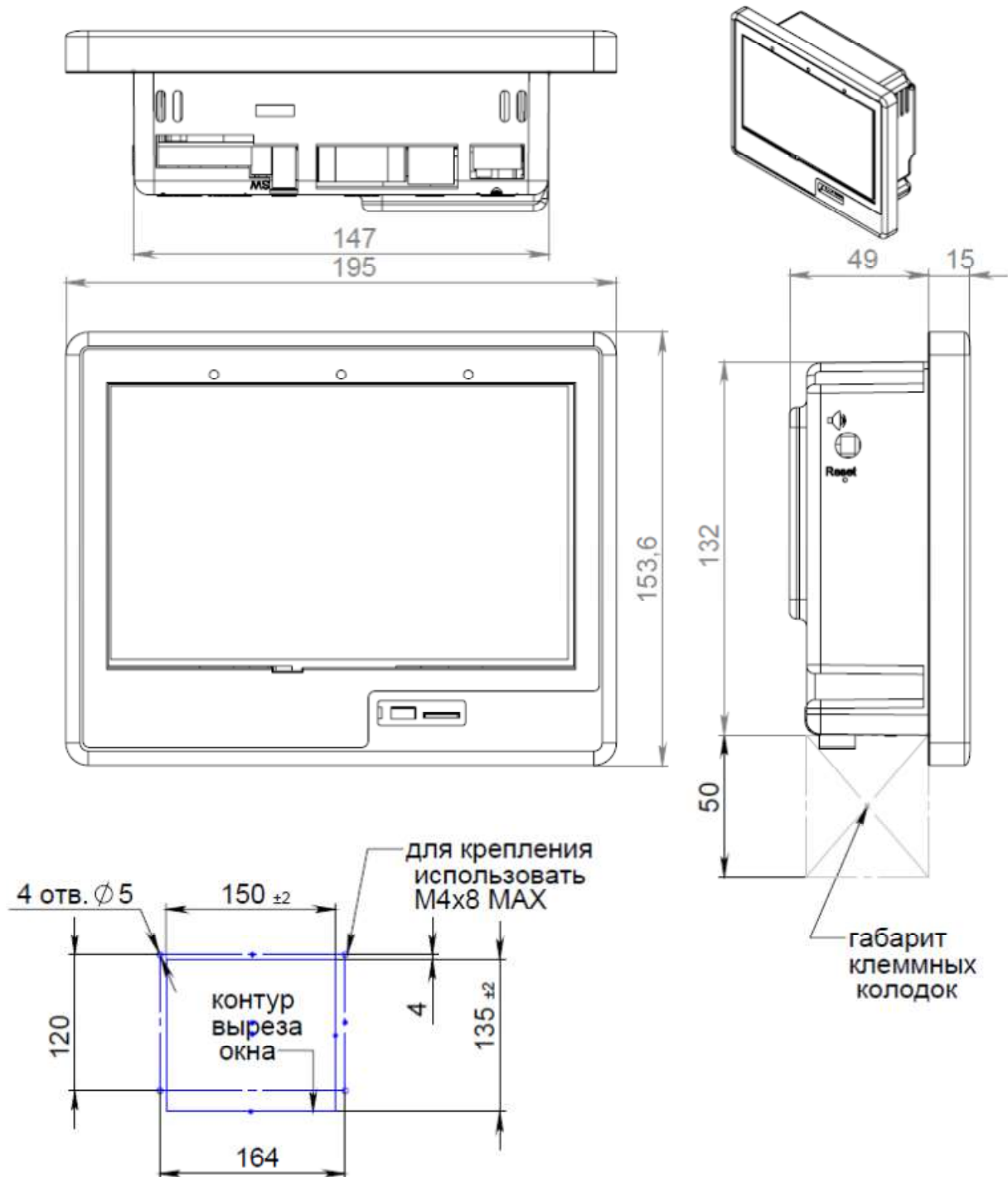
Рисунок 1. Габаритные размеры и размеры выреза в щите АГАВА ПК-50.07
