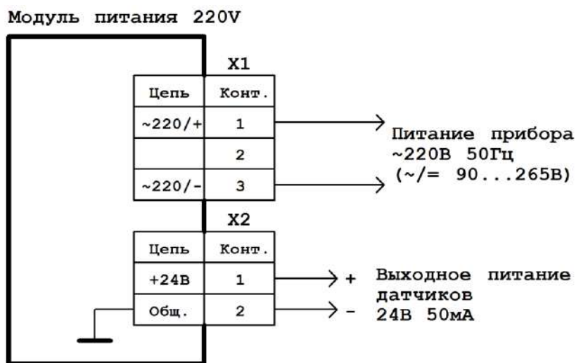
Рисунок 2.6 - Схема подключения модуля 220 V
