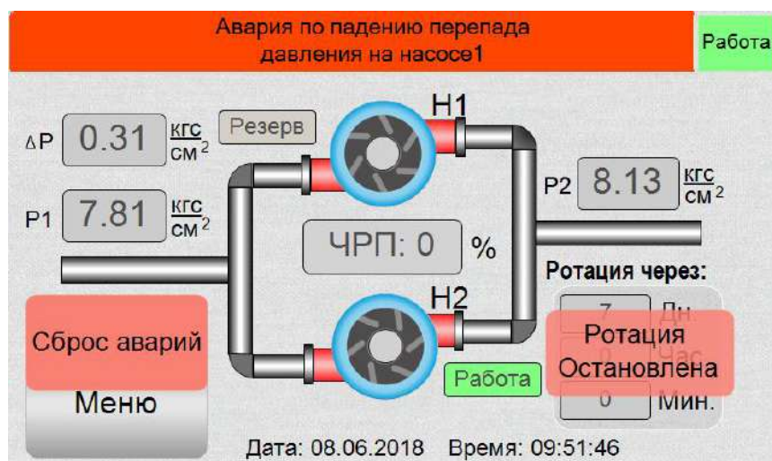
Рисунок 3.23 - Отключение насосов
