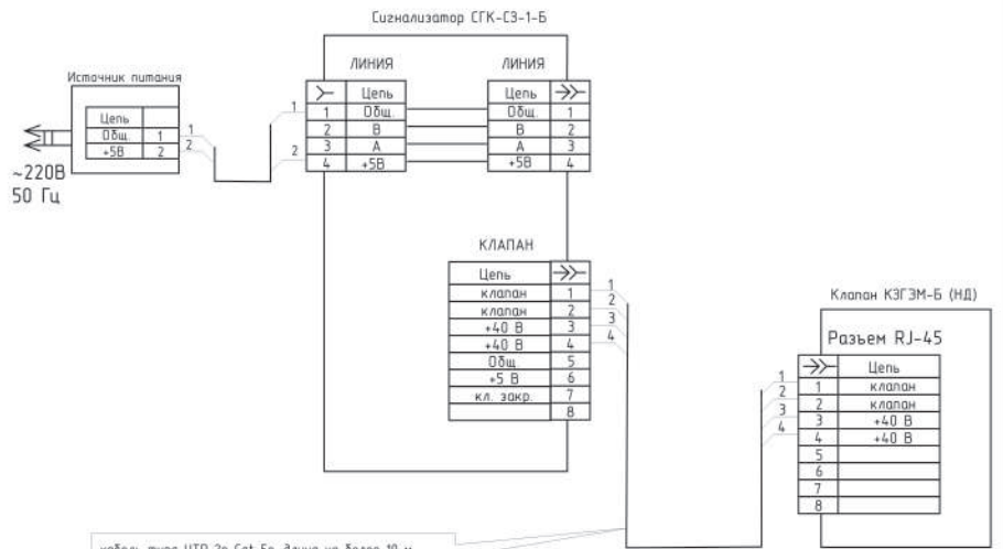
Система автономного контроля загазованности бытовая СГК-1-Б-СН4. Типовая схема соединений.
