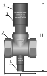
Рисунок 3. – Клапан КЗГЭМ-Б.
