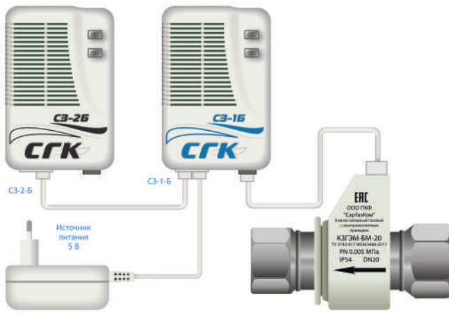
Система автономного контроля загазованности CGK-2-Б с клапаном КЗГЭМ-БМ
