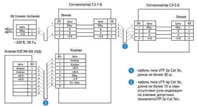
Система автономного контроля загазованности бытовая CGK-2-Б. Типовая схема соединений.
