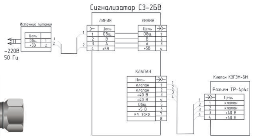
Система автономного контроля загазованности бытовая СГК-1-Б-СО. Типовая схема соединений.
