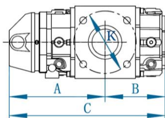
Рисунок Г.1 Габаритные размеры счетчиков газа RABO (G16 – G400 DN100)
